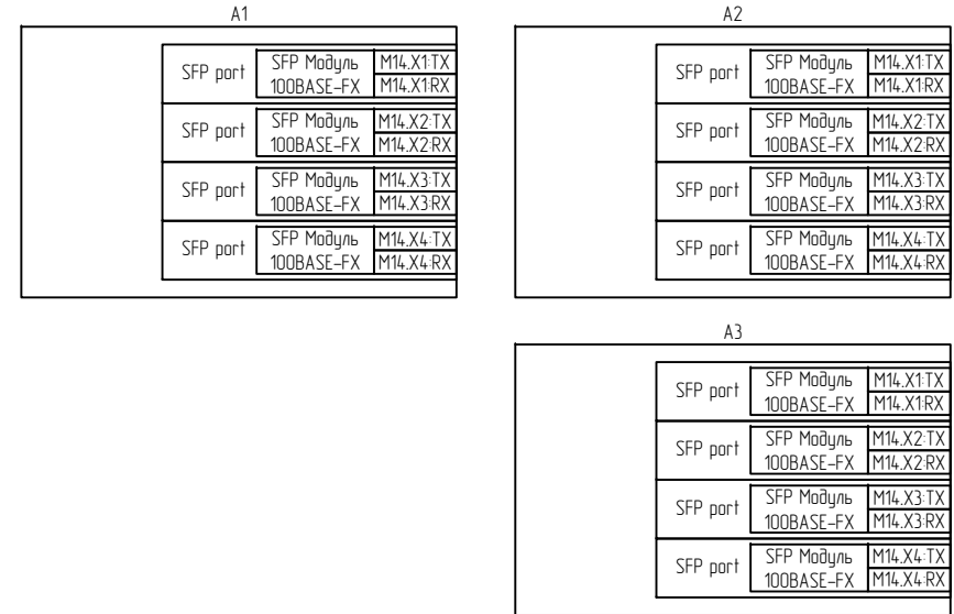
Цепи портов связи терминала
