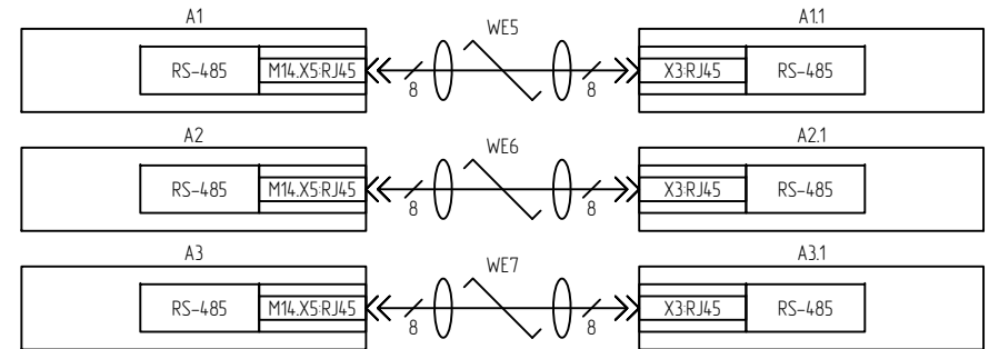
Цепи портов связи терминала с ИЧМ
