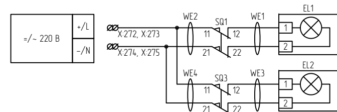
Цепи освещения шкафа
